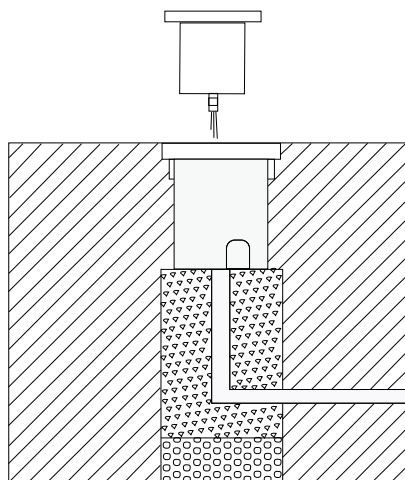
Схема монтажа
